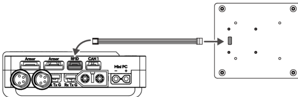
图 3-39 场地交互模块连线示意图
