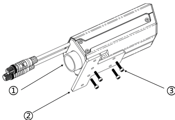
[1] 短枪管 [2] 机器人原有板类零件 1（自制） [3] 螺钉 M2.5
