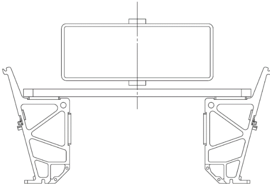
图 3-26 哨兵支撑架安装示意图
