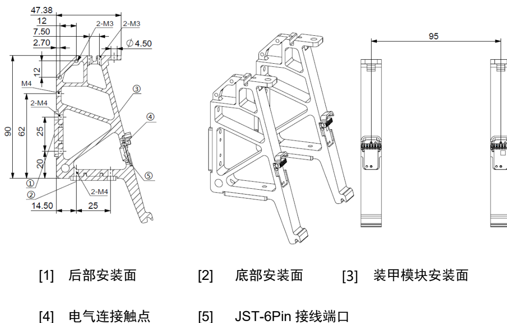
图 3-14 指定装甲支撑架示意图
