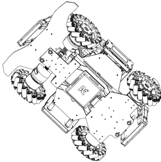
图 3-40 场地交互模块安装示意图
