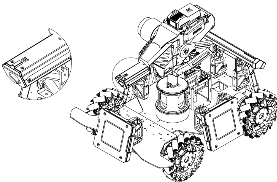
图 3-32 测速模块安装示意图
