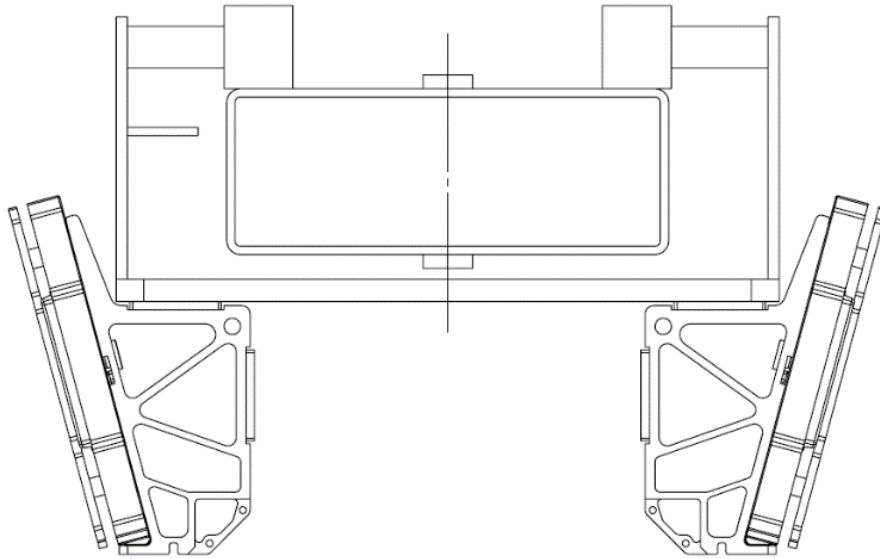
图 3-27 哨兵装甲安装示意图
