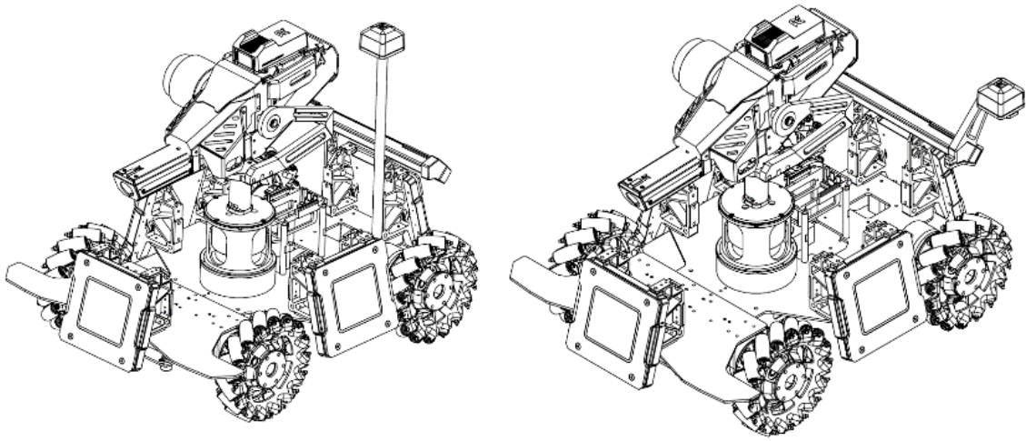
图 3-46 定位模块安装示意图
